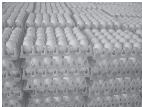
Fig. 5.15: Plastic egg filler flats
