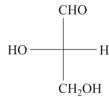
L(-)-ग्लिसरैलिडहाइड
