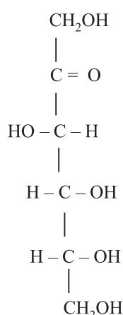
D-फ्रक्टोस
