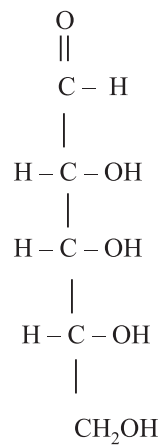
D-राइबोस
