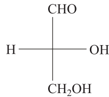
D(+)-ग्लिसरैलिडहाइड
