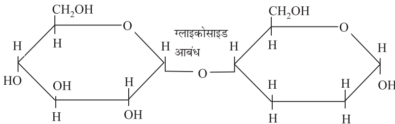
माल्टोस
