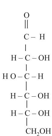
D-ग्लूकोस
