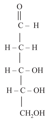
2-डि-ऑक्सी-D-राइबोस
